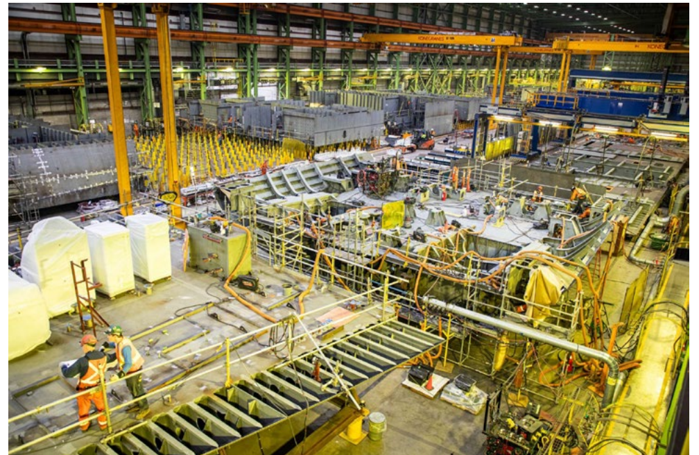
Le futur NCSM Fraser en construction à Irving Shipbuilding à Halifax.
